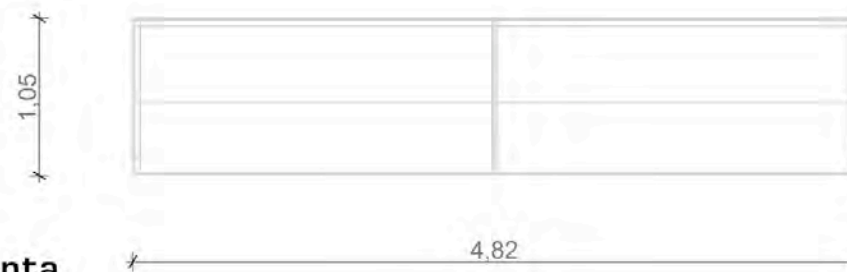
Planta
