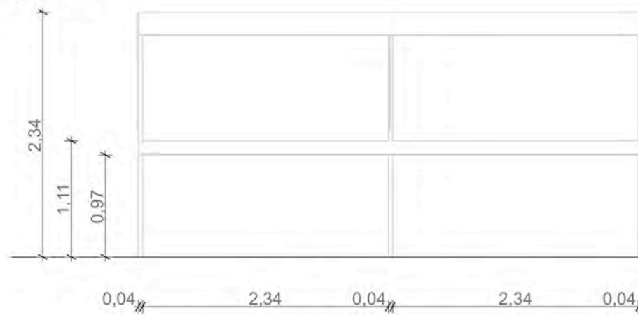
Alzado
