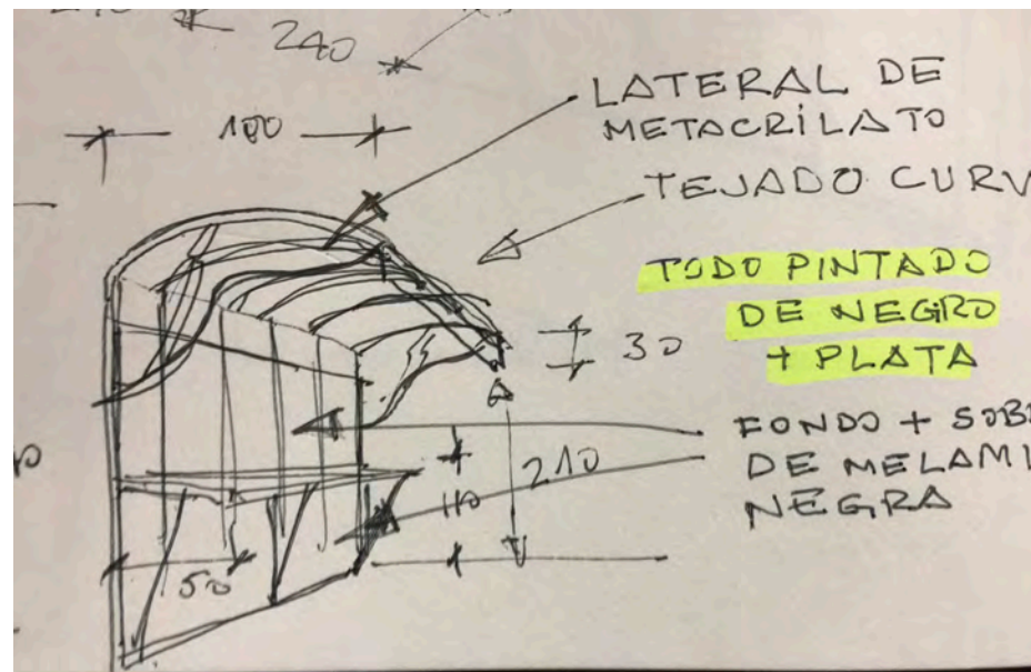
Alzado
